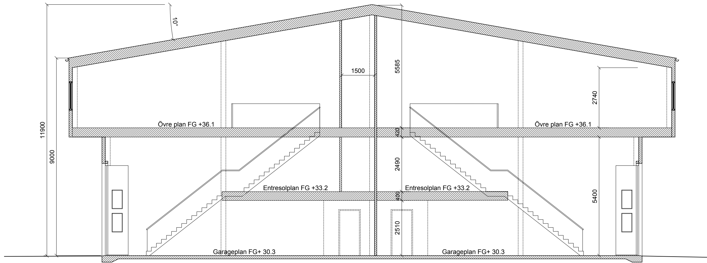
Principsektion A-A HUS A+B
